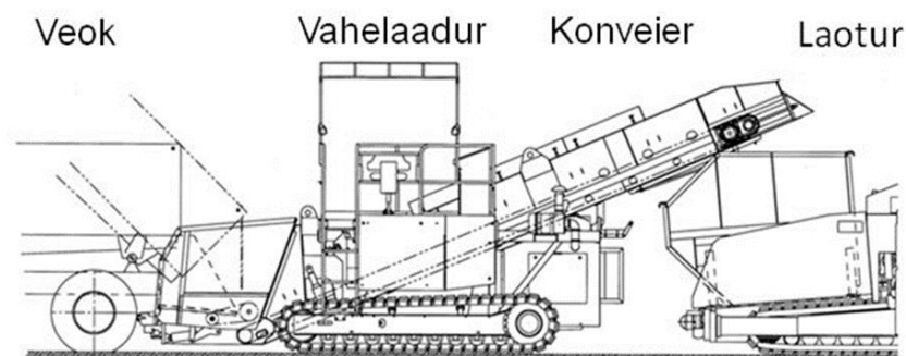
Joonis 59 Kasutatava tehnika põhimõtteskeem 28
