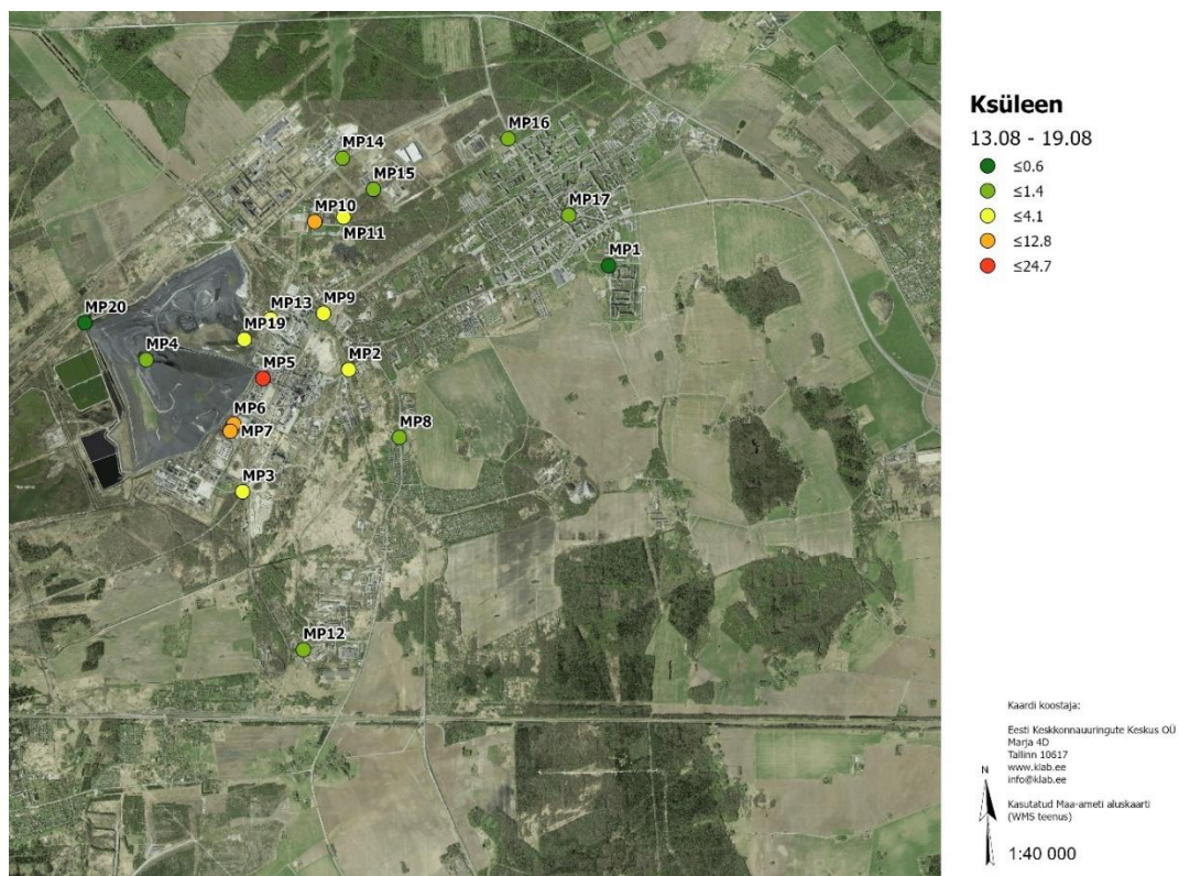
Joonis 49 Ksüleeni nädalakeskmine kontsentratsioon, 13.08 – 19.08.24
