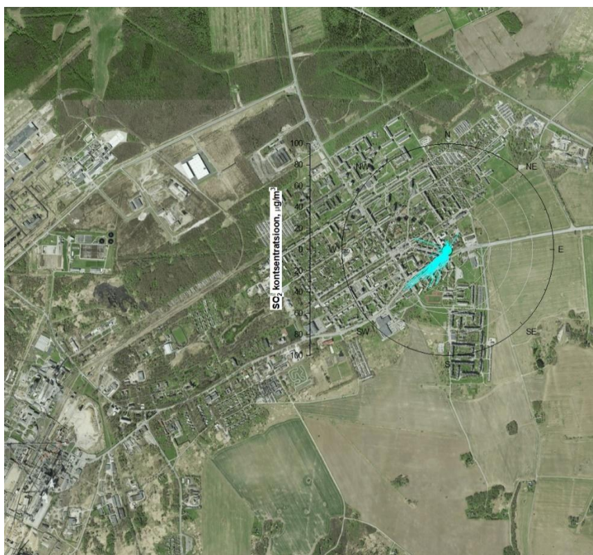
Joonis 66 SO 2 kontsentratsiooniroos, Mobair-1 mõõtepunkt
