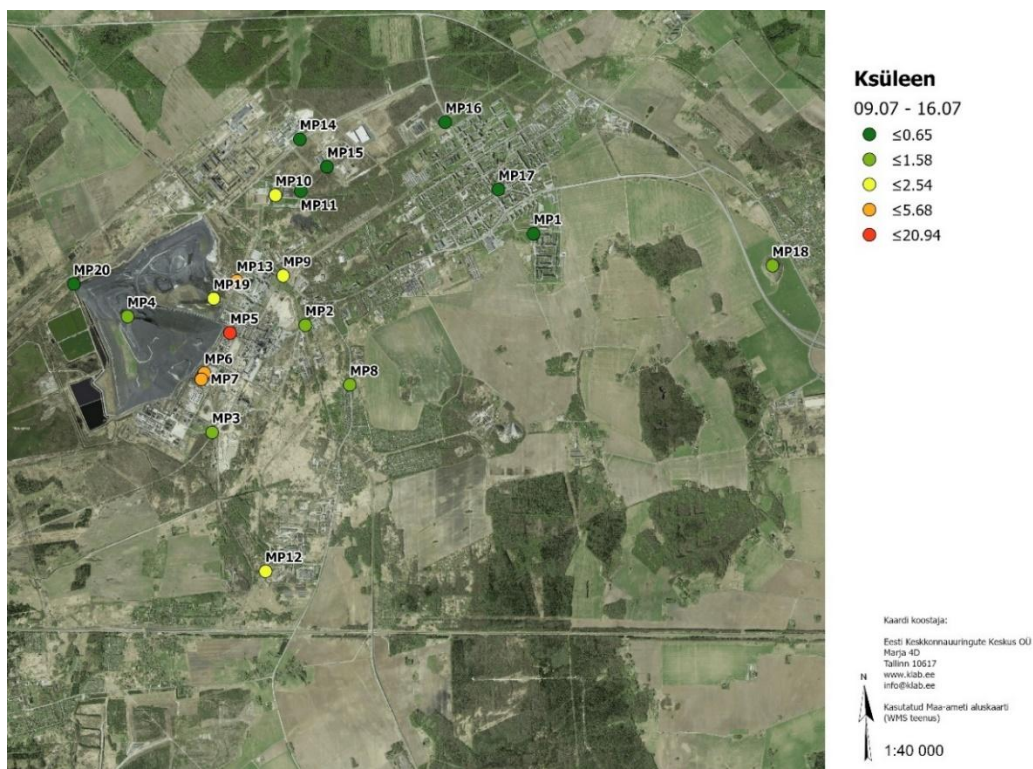
Joonis 48 Ksüleeni nädalakeskmine kontsentratsioon, 09.07 – 16.07.24
