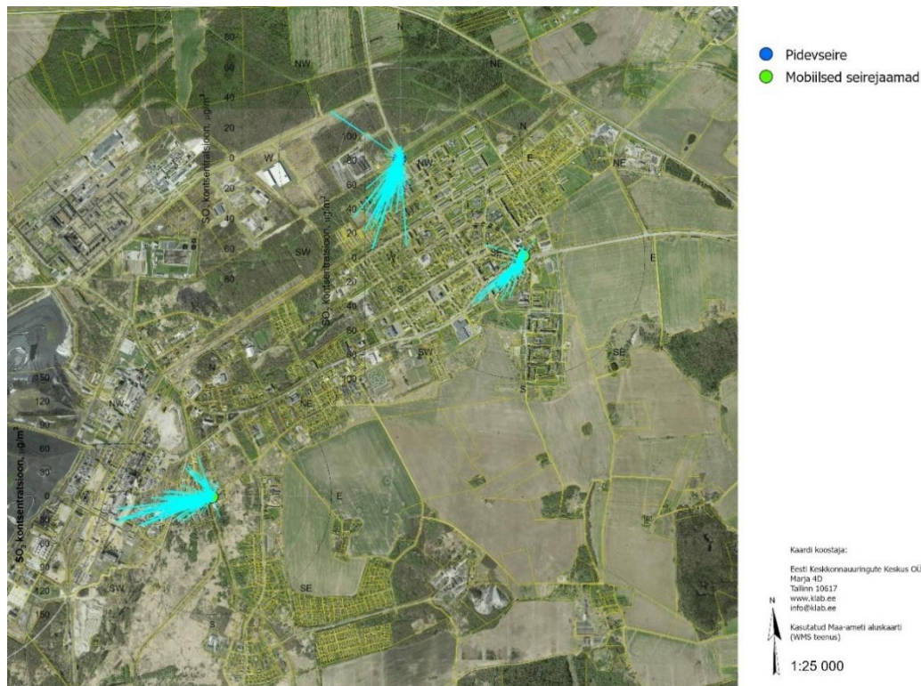
Joonis 111 SO 2 kontsentratsiooniroosid Mobair-1 ja Mobair-2 mõõtepunktides ning Kohtla-Järve seirejaamas
