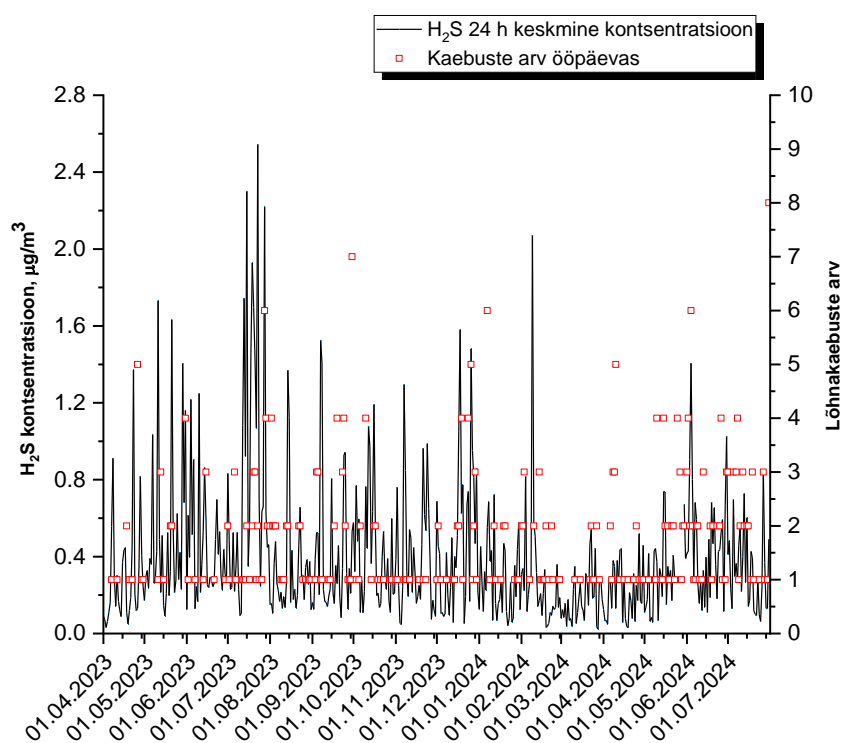
Joonis 30 H 2 S 24 h keskmine kontsentratsioon Kohtla-Järve seirejaamas ning kaebuste arv ööpäevas
