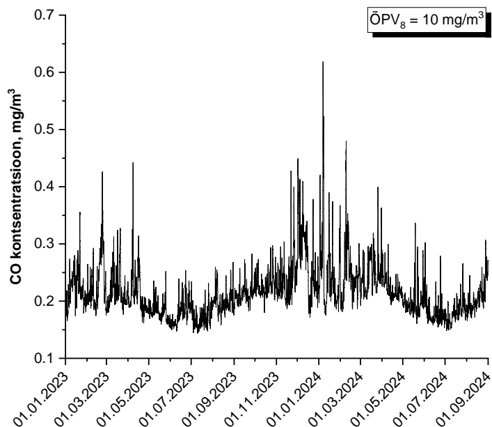
Joonis 126 CO 8 h keskmine kontsentratsioon, Kohtla-Järve seirejaam
